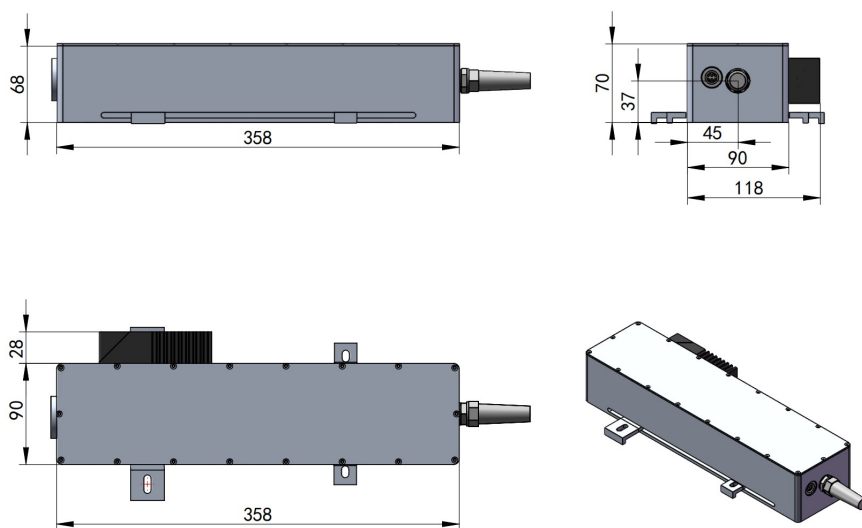
机箱尺寸图
