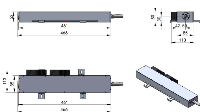
激光头尺寸图
