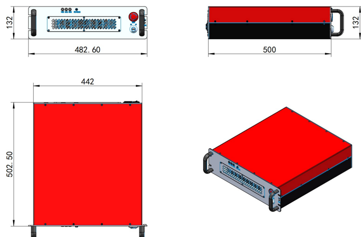
机箱尺寸图
