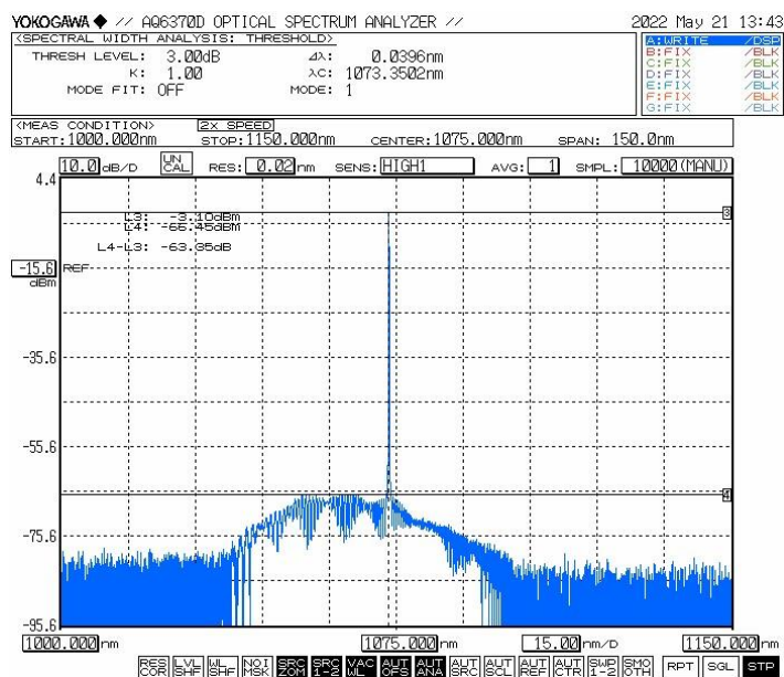
光谱测试图
