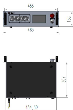
机箱尺寸图-风冷
