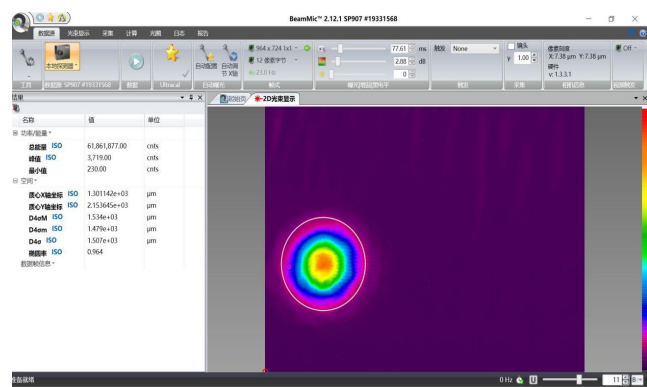
光斑测试图
