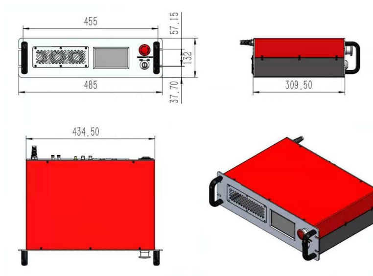
机箱尺寸图
